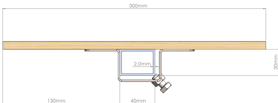
Figuur 4: Vooraanzicht van een plateau met bevestigingsbeugel
