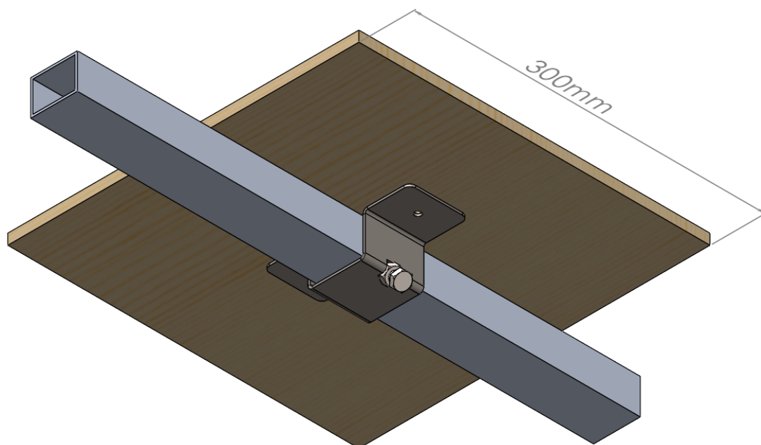
Figuur 3: Vooraanzicht van een plateau met bevestigingsbeugel
