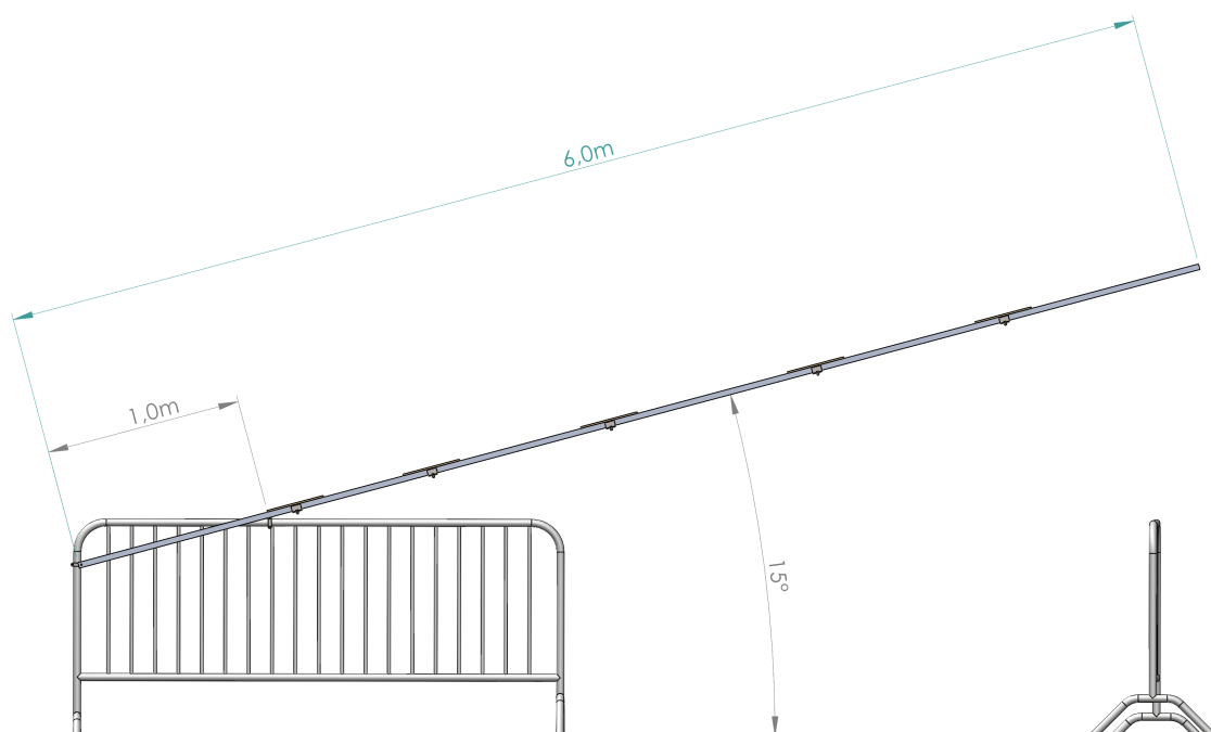
Figuur 2: Zijaanzicht van de wedstrijd baan
